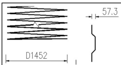
图6 钢筋笼简易构造图(尺寸mm)
