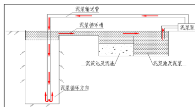
图 2 换浆法正循环清孔原理图
