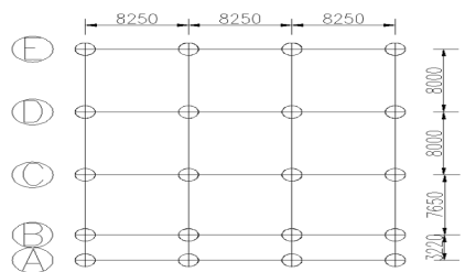
图 3 单排架桩基平面布置图
