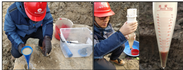
图7 泥浆粘度检测
