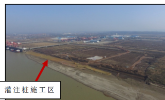
图 1 嵌岩灌注桩施工现场
